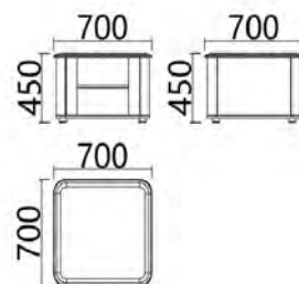
奧瑾 F1307 方几
