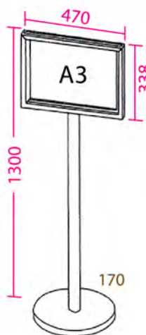
直立式提示牌 Sign Stand
